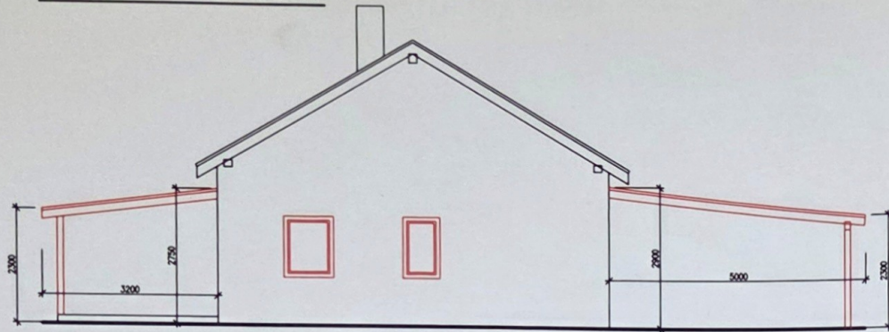
POHLED VÝCHODNÍ
