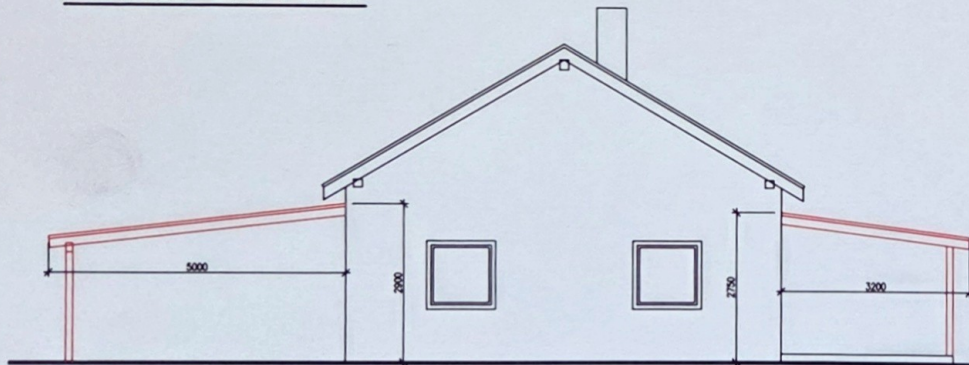
POHLED ZÁPADNÍ
